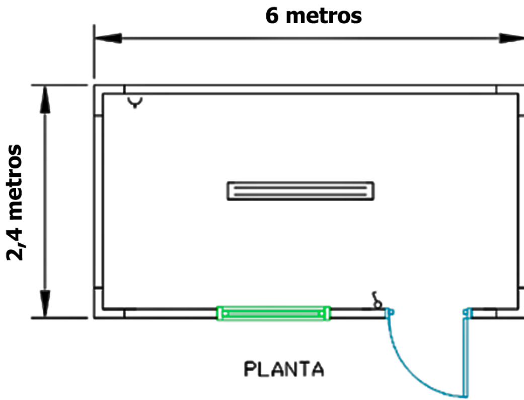
Plano y medidas de la caseta
