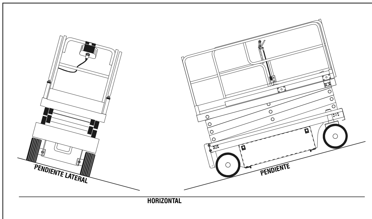
Figura 4-1. Pendiente y pendiente lateral
