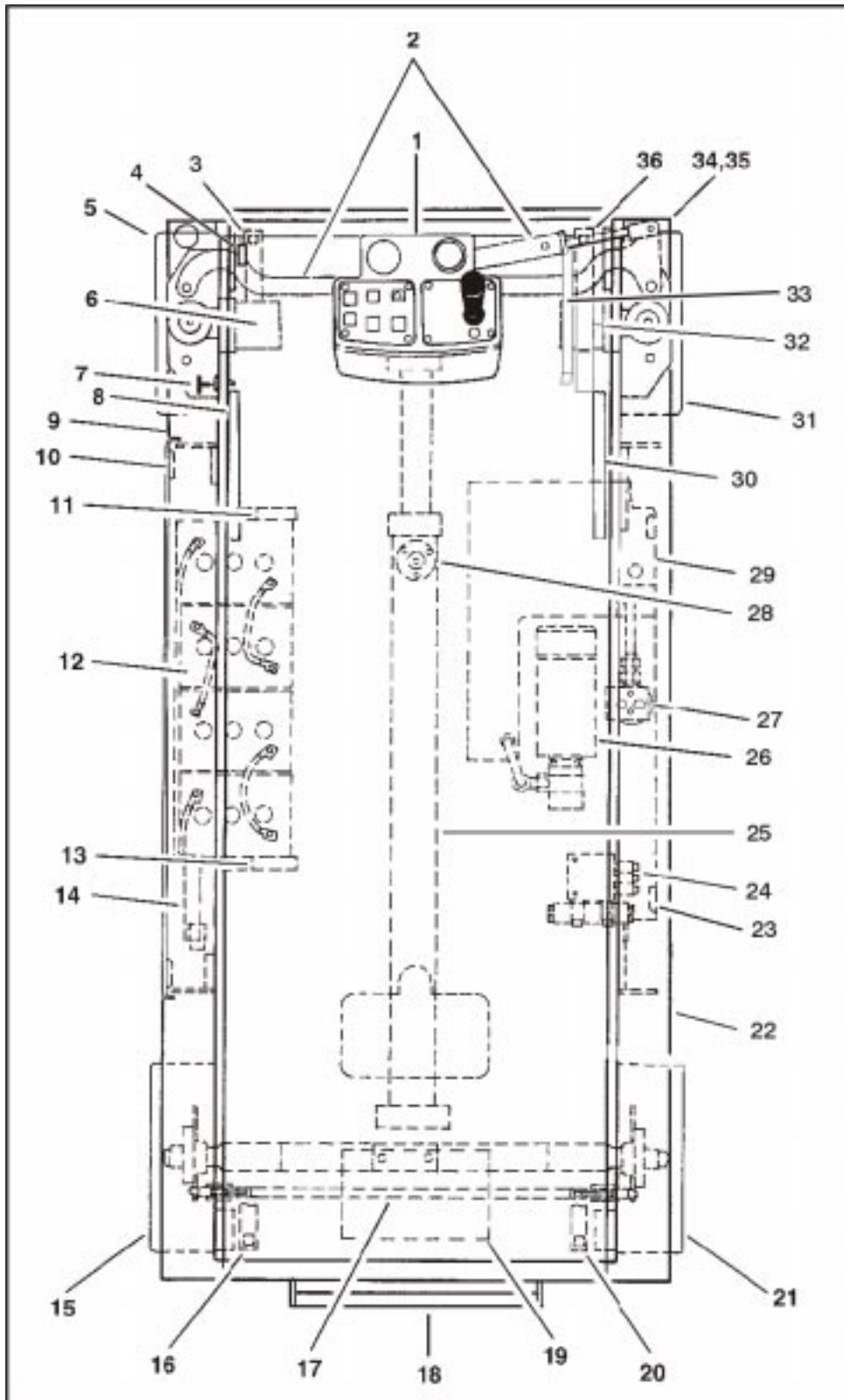
Figura 2-2. Diagrama de inspección visual diaria (hoja 1 de 3)
