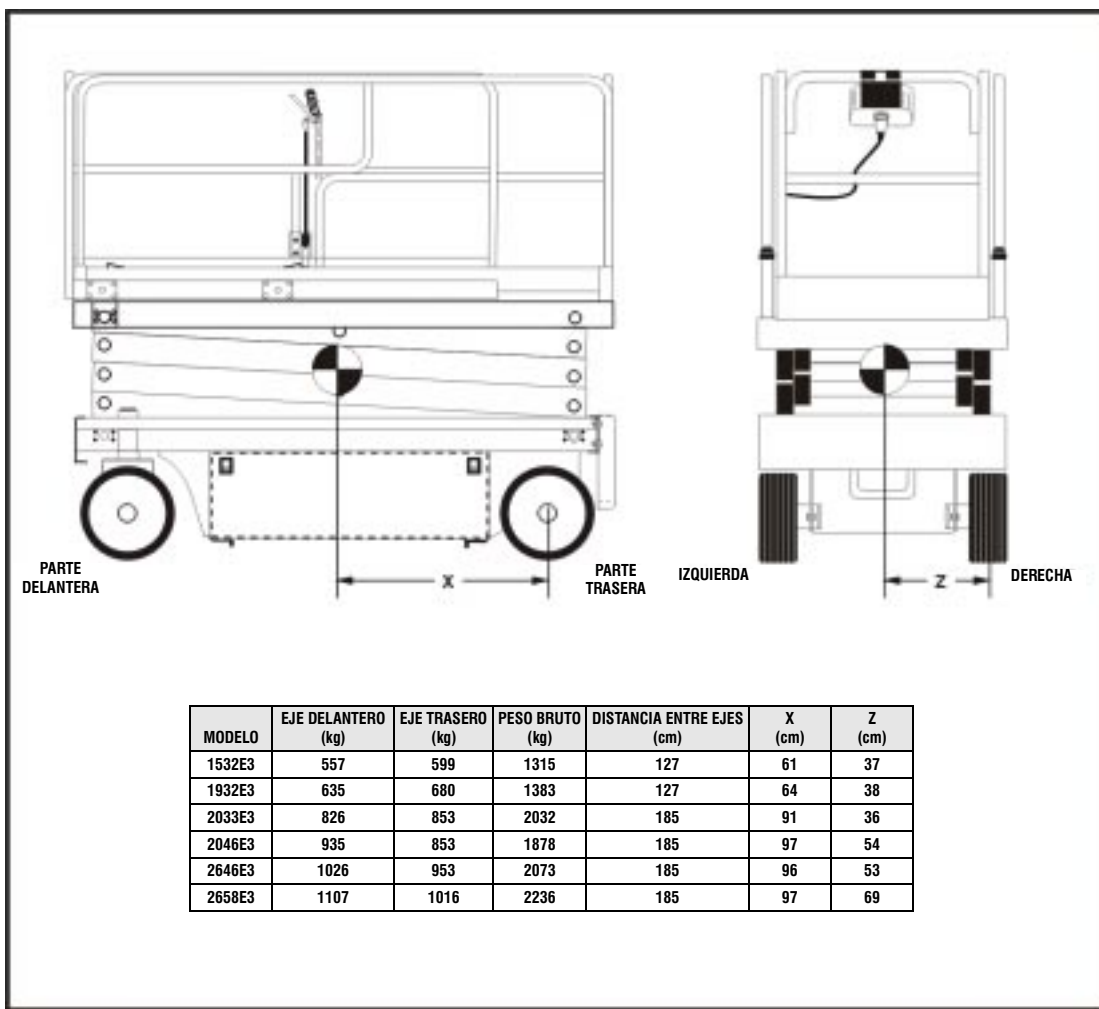
Figura 4-3. Tabla de levante
