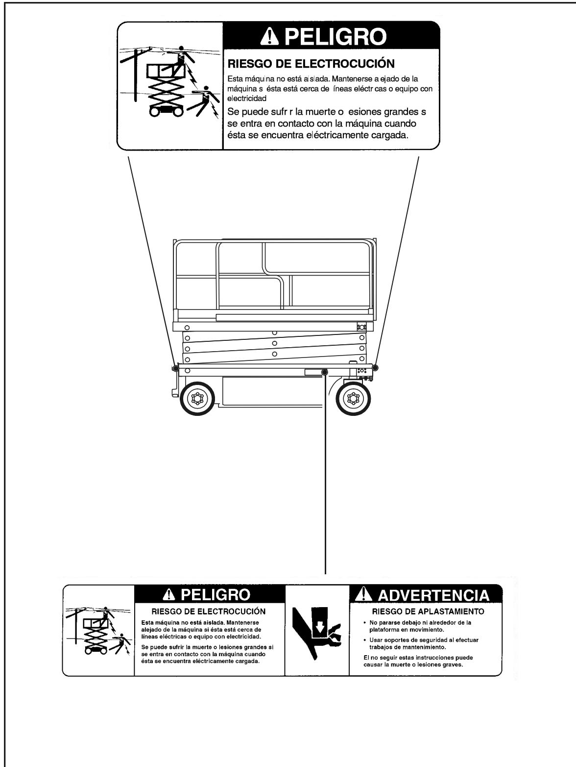
Figura 3-6. Ubicación de etiquetas (lado derecho)
