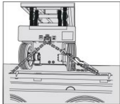
Figura 4-2. Amarre de modelo E3 (configuración típica en partes delantera y trasera)
