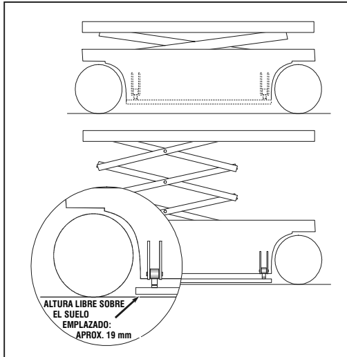
Figura 2-1. Funcionamiento del sistema protector contra baches
